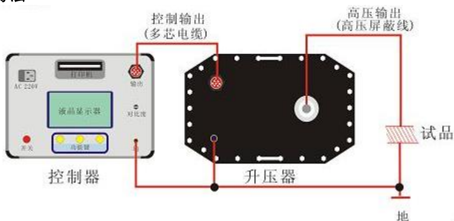
图 4 (连线图)
