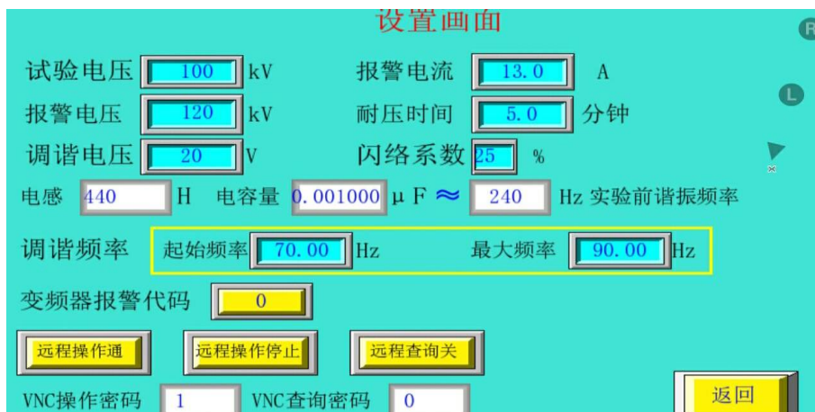
试验前谐振频率计算结果值图 2-12
