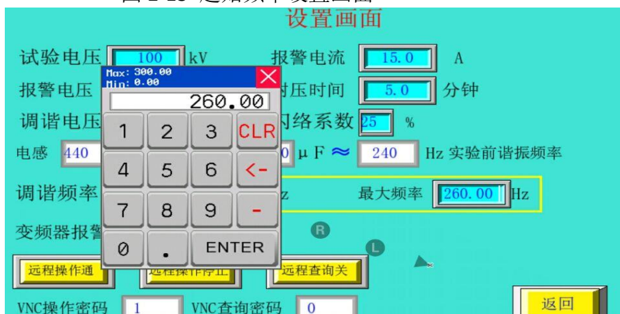
图 2-14 最大频率设置画面
