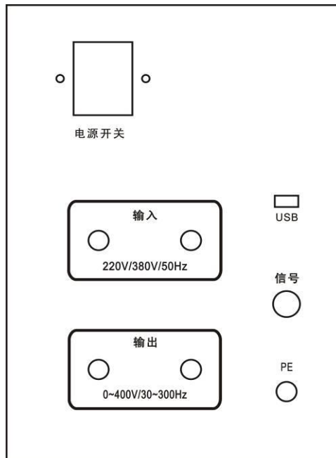
图1-2 侧面接线图
