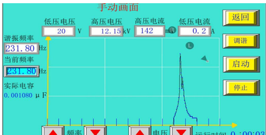
图 4-3 手动模式自动调谐画面
